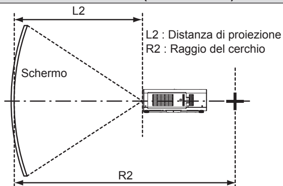
ARCO VERTICALE (Vista laterale)
