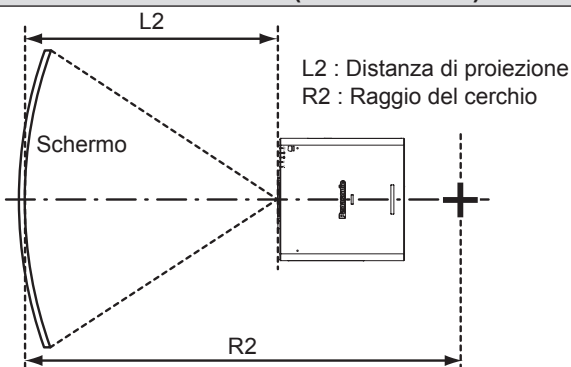
ARCO ORIZZONTALE (Vista dall'alto)
