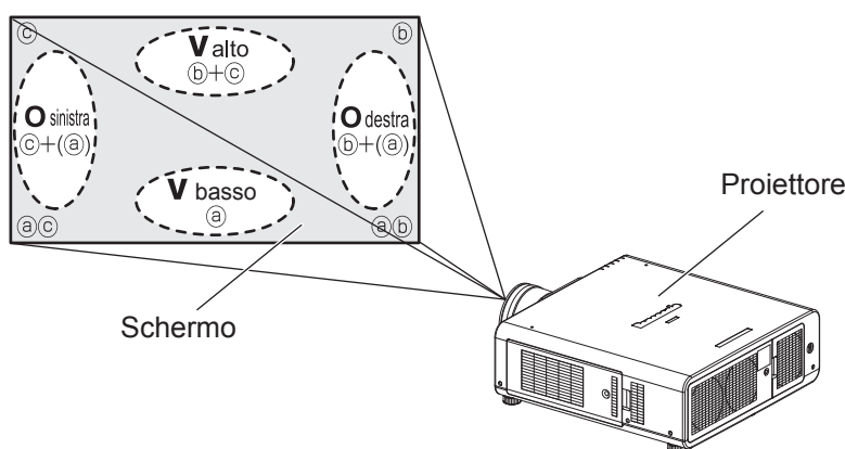
Figura 3 : Relazione tra ubicazione di regolazione e vite di regolazione
