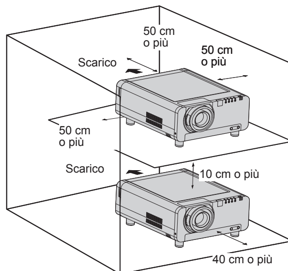
(Figura 2: dimensioni in caso di utilizzo di due unità)
