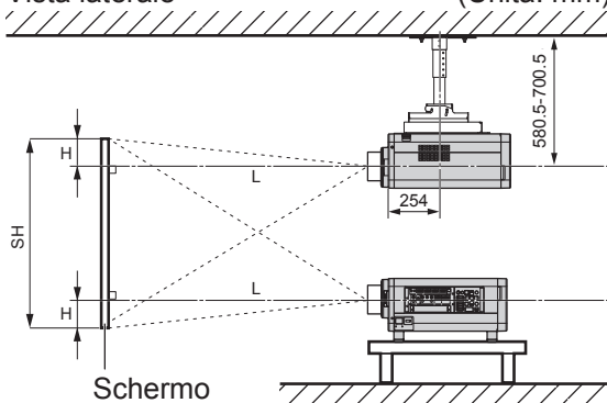
Vista laterale (Unità: mm)
