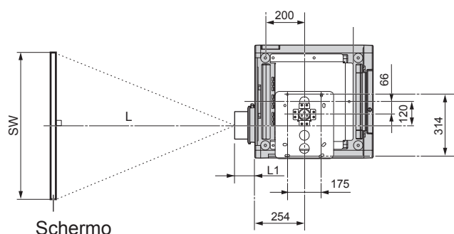
(Unità: mm)
